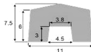
► Plaques compatibles avec les poteaux rainurés réversibles en démoulage différé de nos autres clôtures écran
