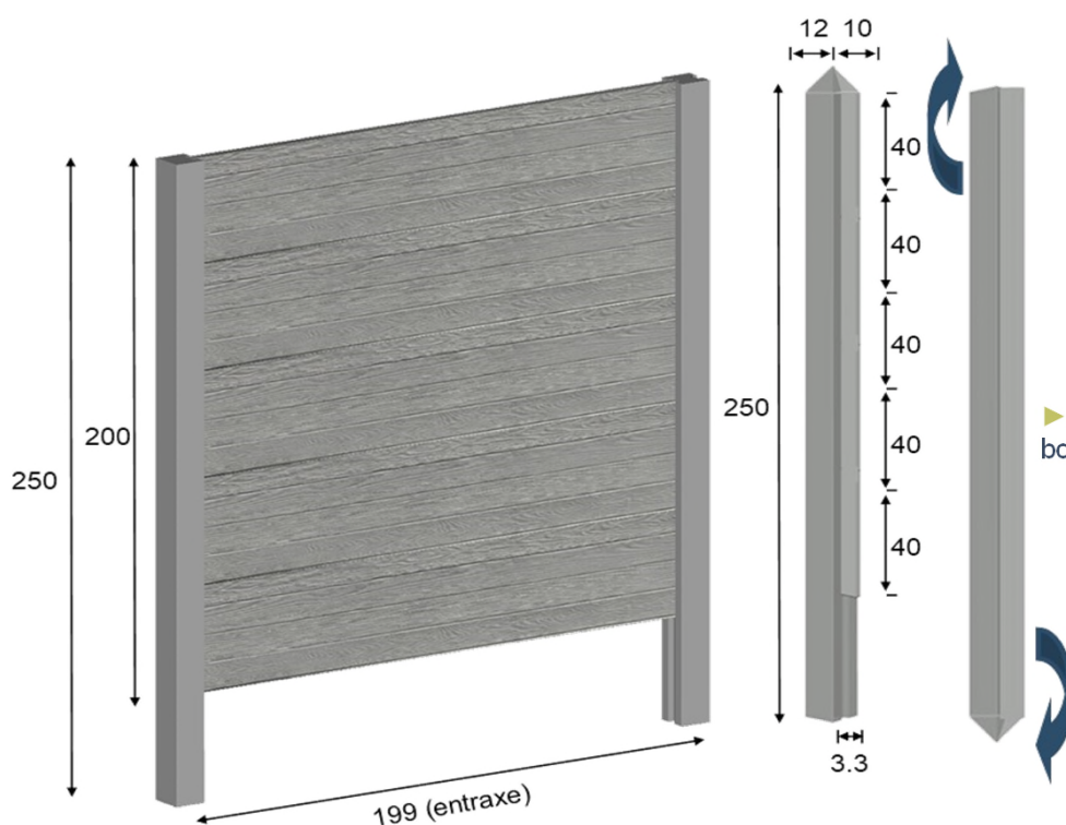
► Poteau réversible avec au choix une finition pointe de diamant ou une finition plate
