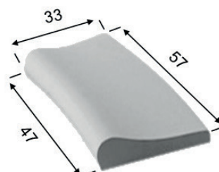
MARGELLE SABLÉE GALBÉE COURBE RAYON 150
