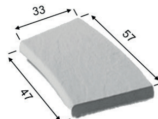
MARGELLE ARDOISÉE PLATE COURBE RAYON 160
